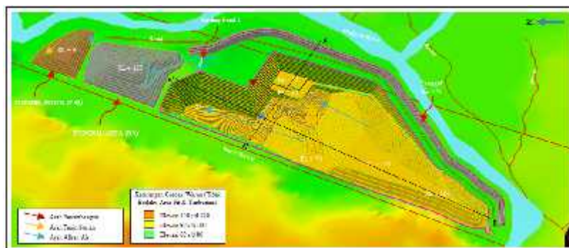
Gambar 15. Peta Kemajuan Tambang Tahun ke – 7
